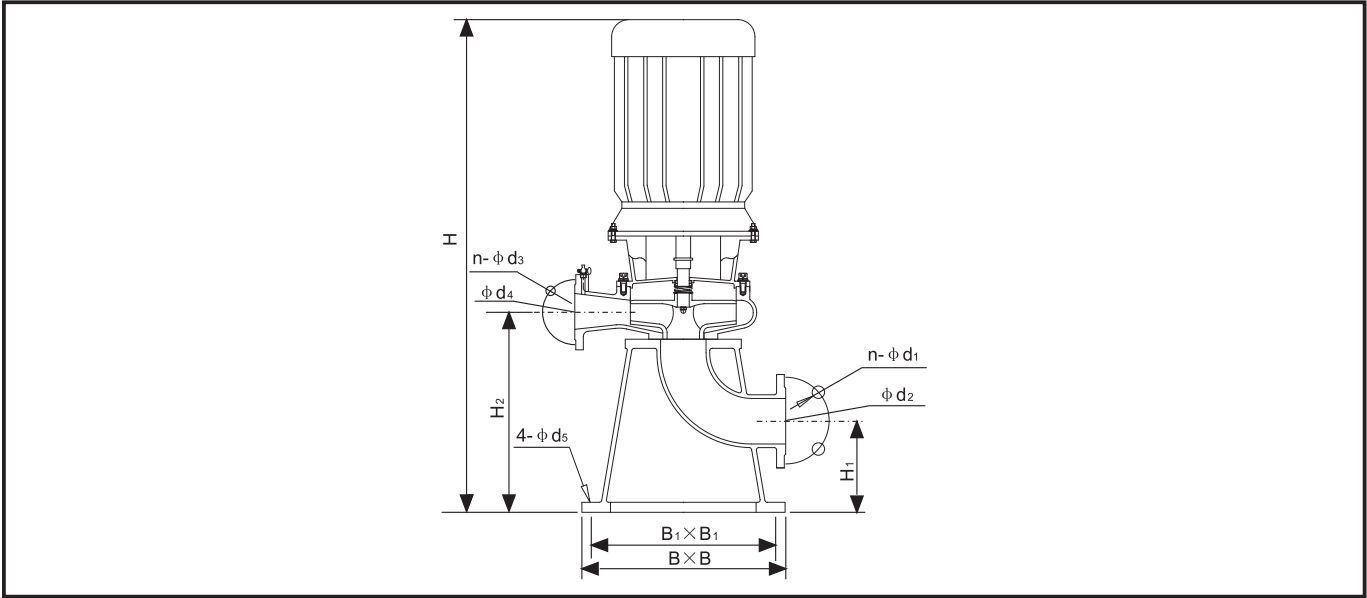
外形尺寸图
